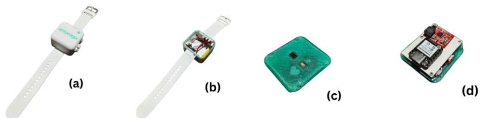
Gambar 4. 1 Prototipe ANTARAGA: (a) tampak atas, (b) tampak dalam, (c) tampak bawah, (d) susunan komponen
